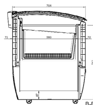
Skalldyr innsats m/bunnrist
